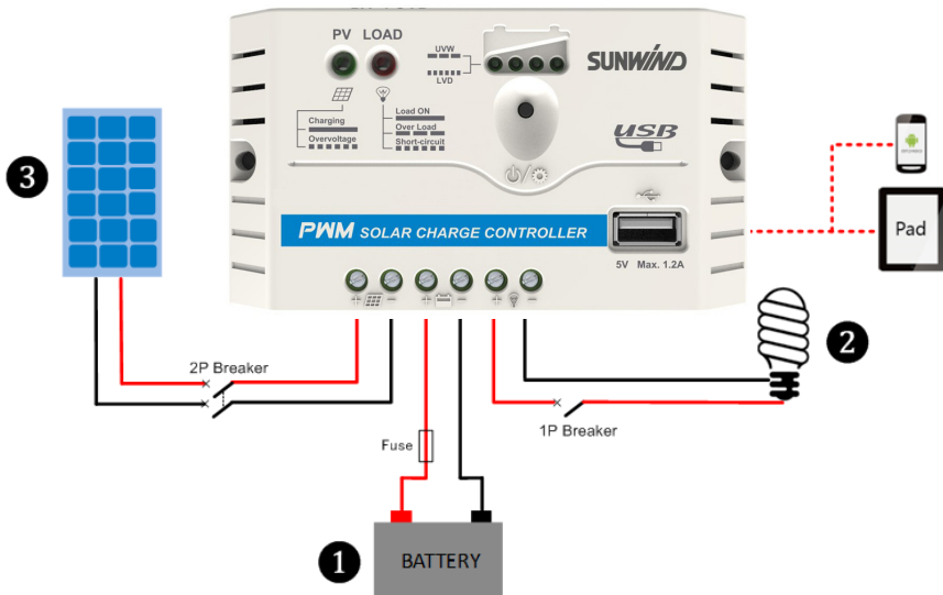
Kuva 2 – Liitäntä
